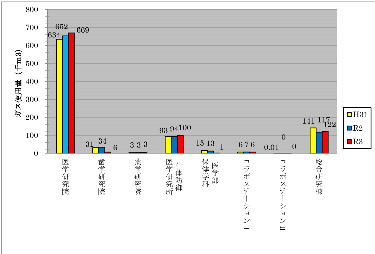
【グラフ5 建物別ガス使用量】
