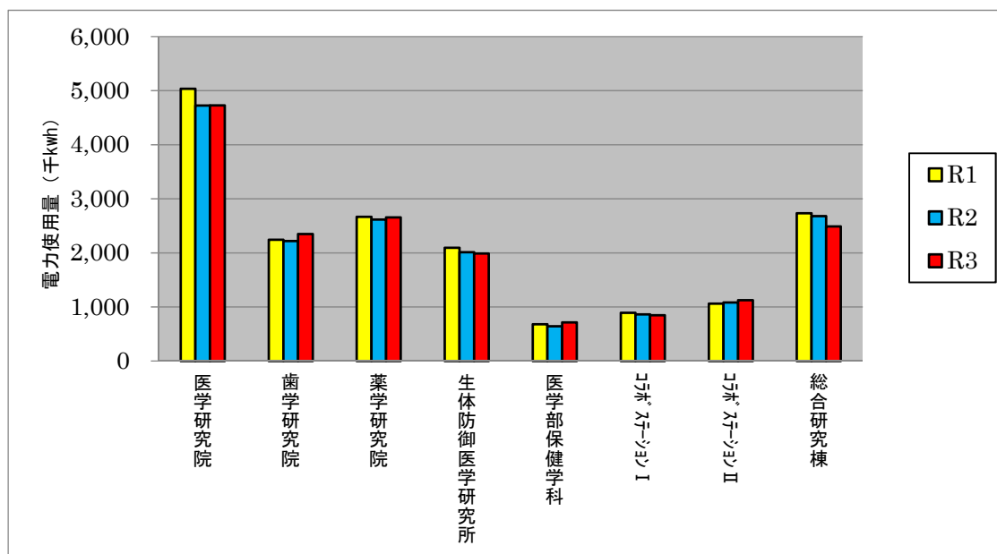
【グラフ3 部局・建物別電力使用量】
